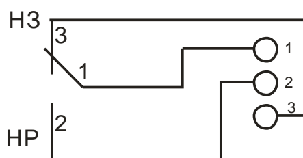
Рисунок Б.1 - Исполнение с гермовводом, исполнение с кабельным вводом G1-A
