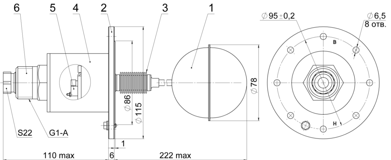
Рисунок А.2 - Исполнение с кабельным вводом G1-A
